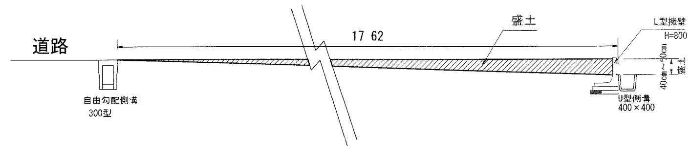
標準断面図
